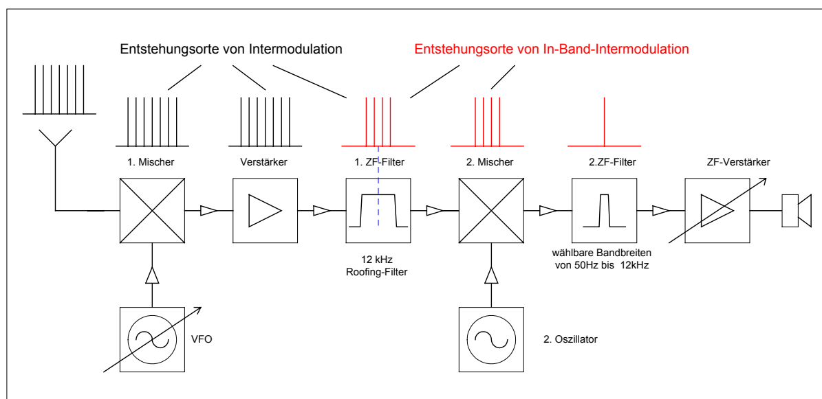
Bild 1: Prinzipschaltbild eines Doppelsuperhet mit Vorselektion in der 1.ZF und endgültiger Selektion der in 2. ZF/DSP
