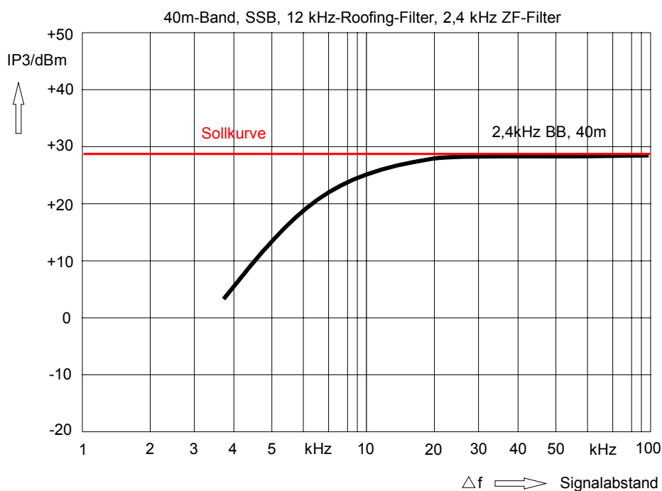
Bild 3: IP 3 in Abhängigkeit vom Signalabstand
