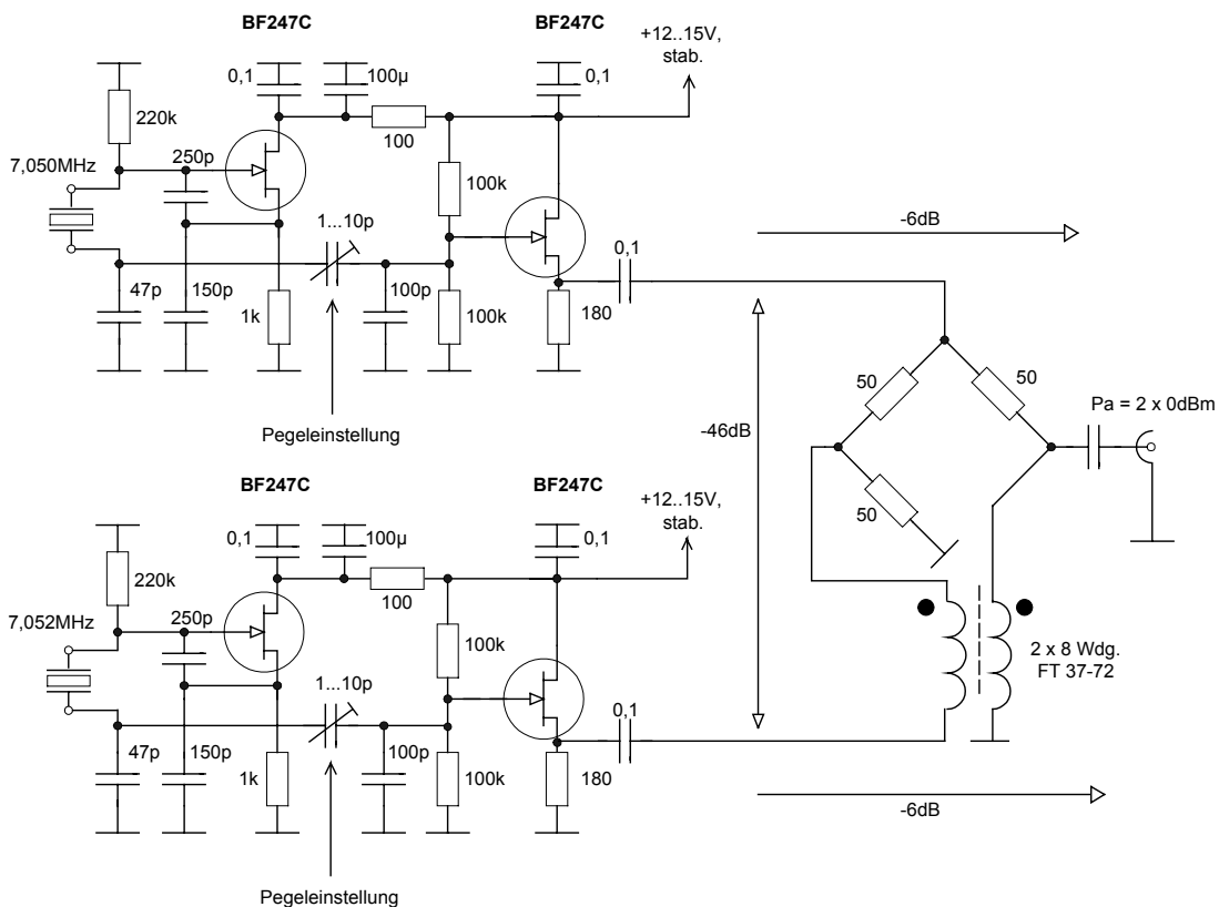
Bild 10: Schaltung eines geeigneten Doppeltongenerator für 1-30 MHz
